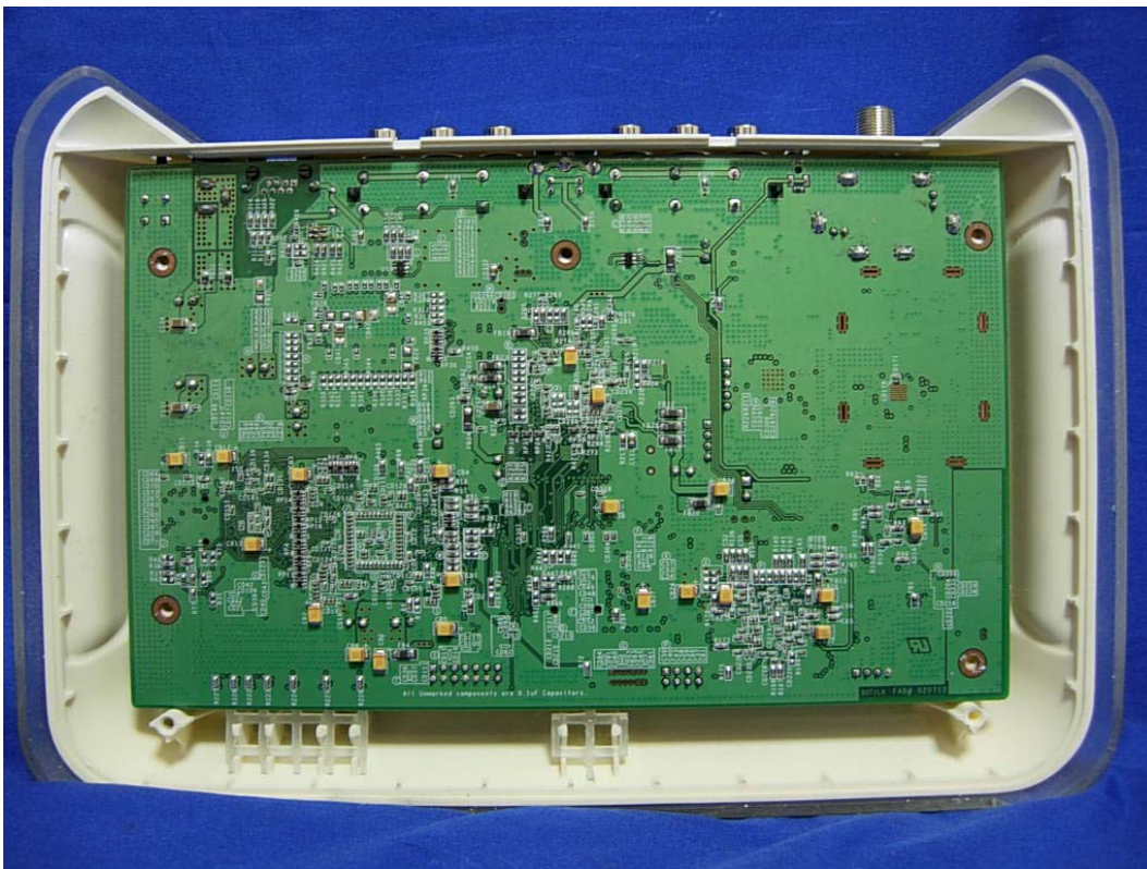
(5) EUT Photo
