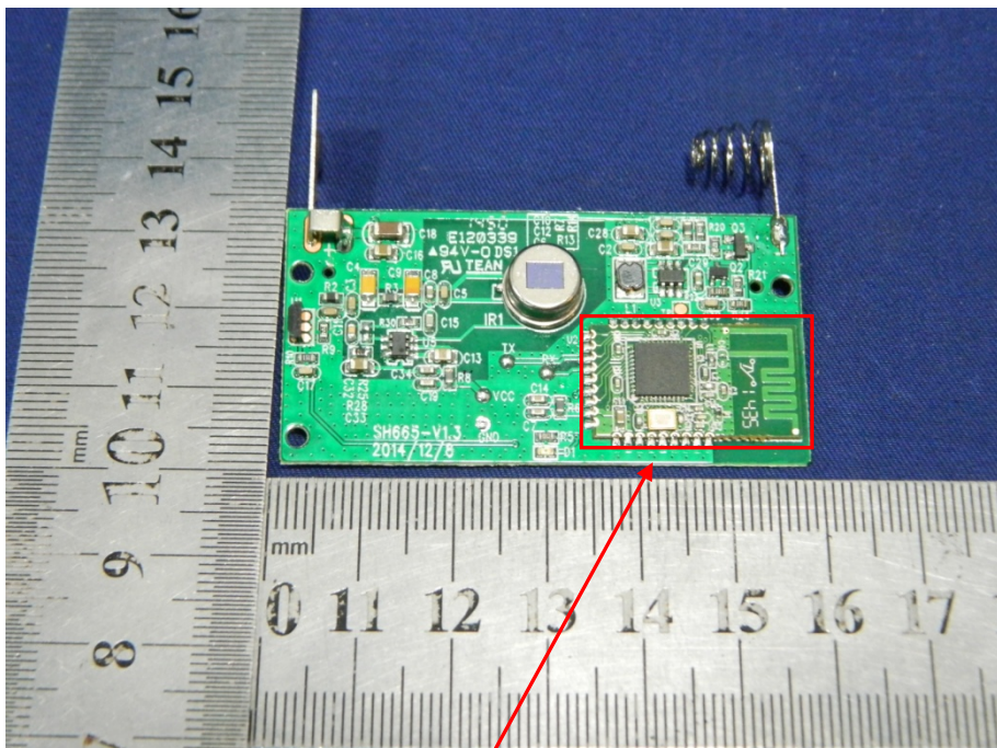
Zigbee Module
