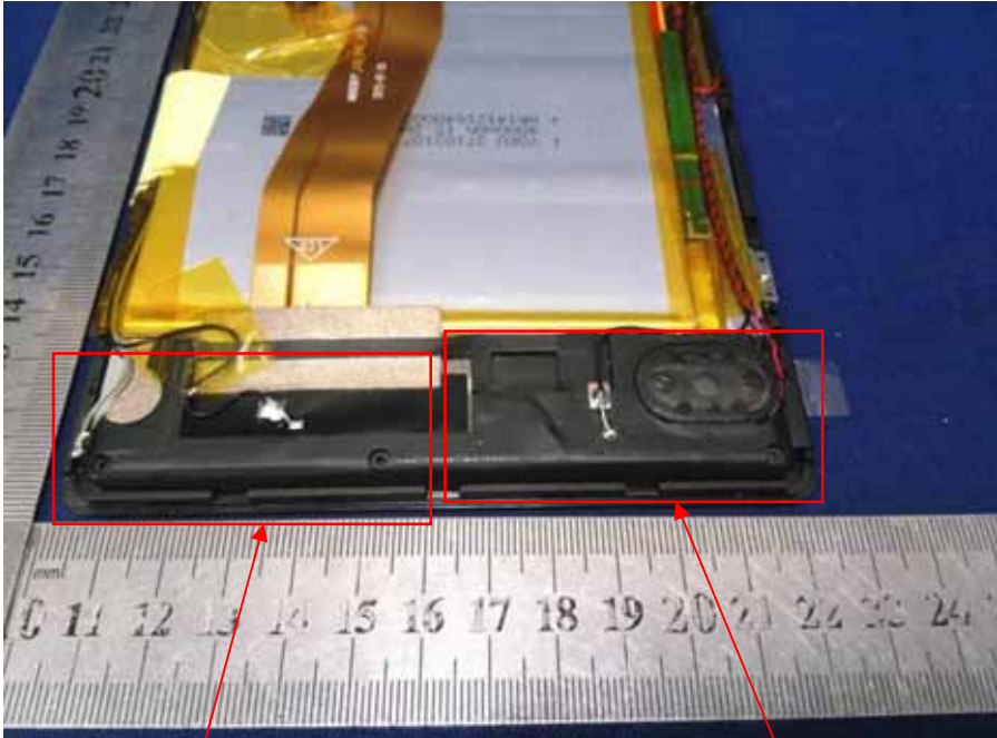
4G Antenna/Main Antenna
