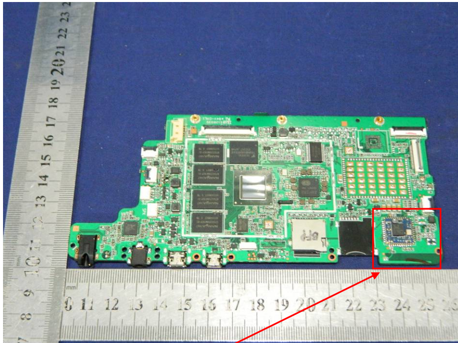
Bluetooth Module
