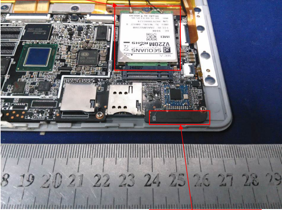
Bluetooth/Wifi Antenna
