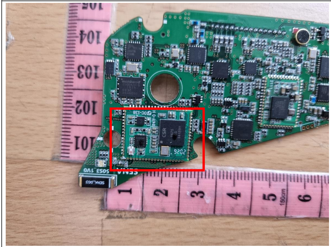
BT module
