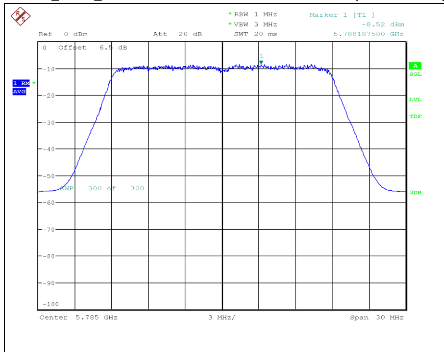
802.11n_HT20 _ ch.157
