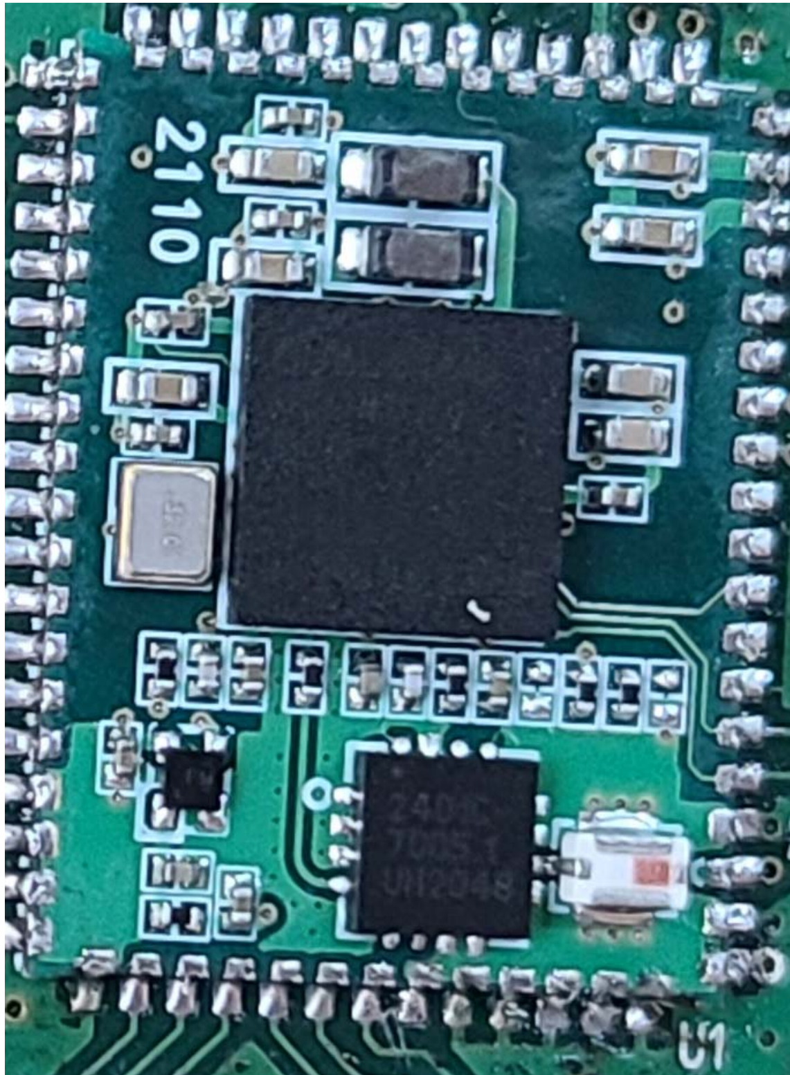
BT Module
