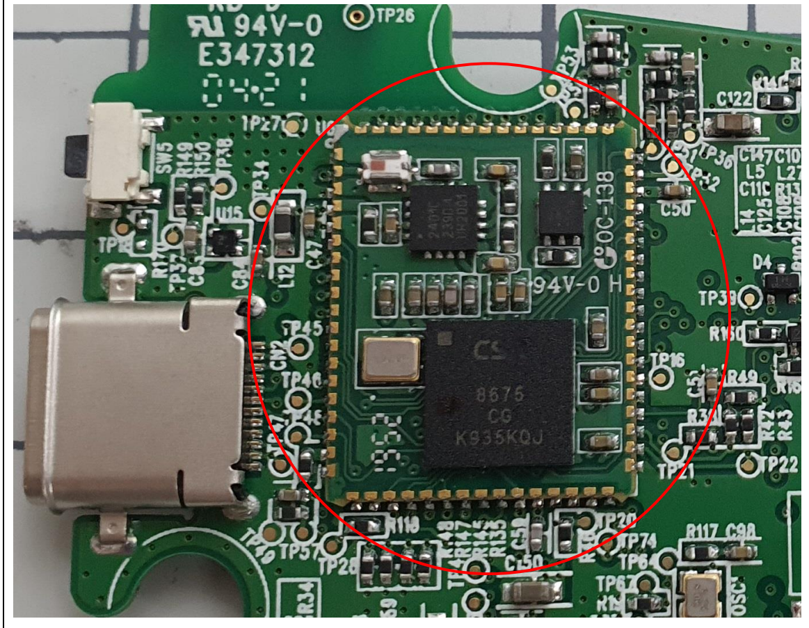
BT Module
