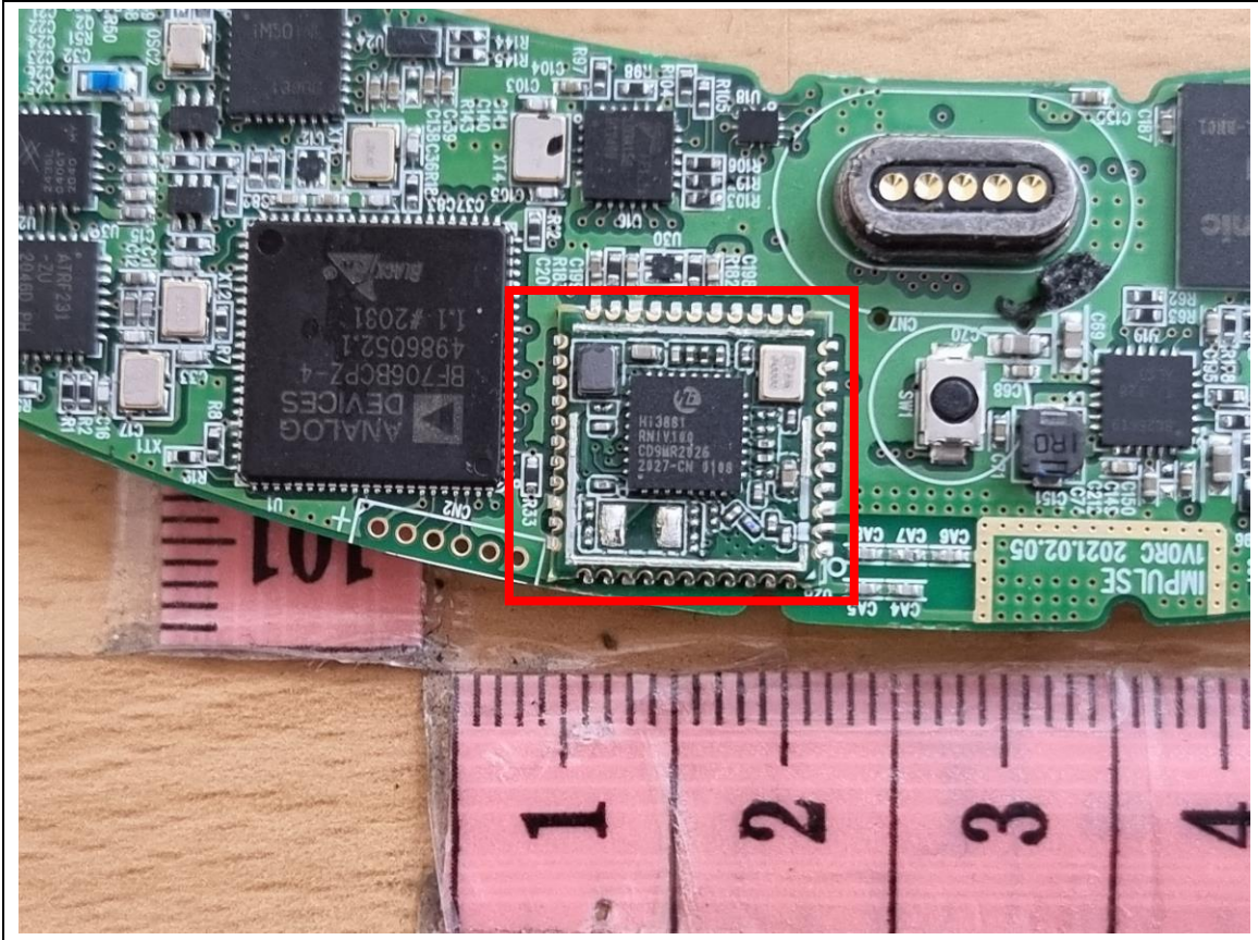
WLAN Module
