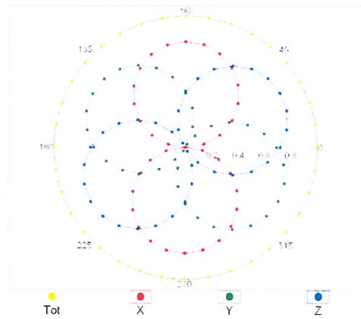
f=1800 MHz,R22
