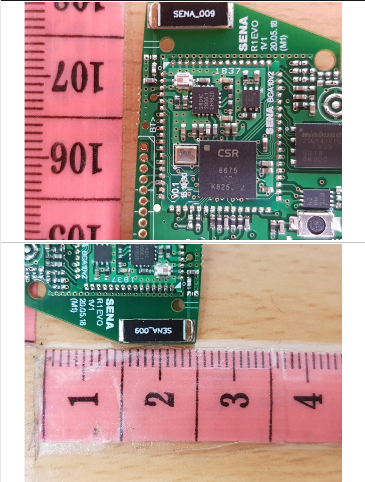
Bluetooth Module & Antenna
