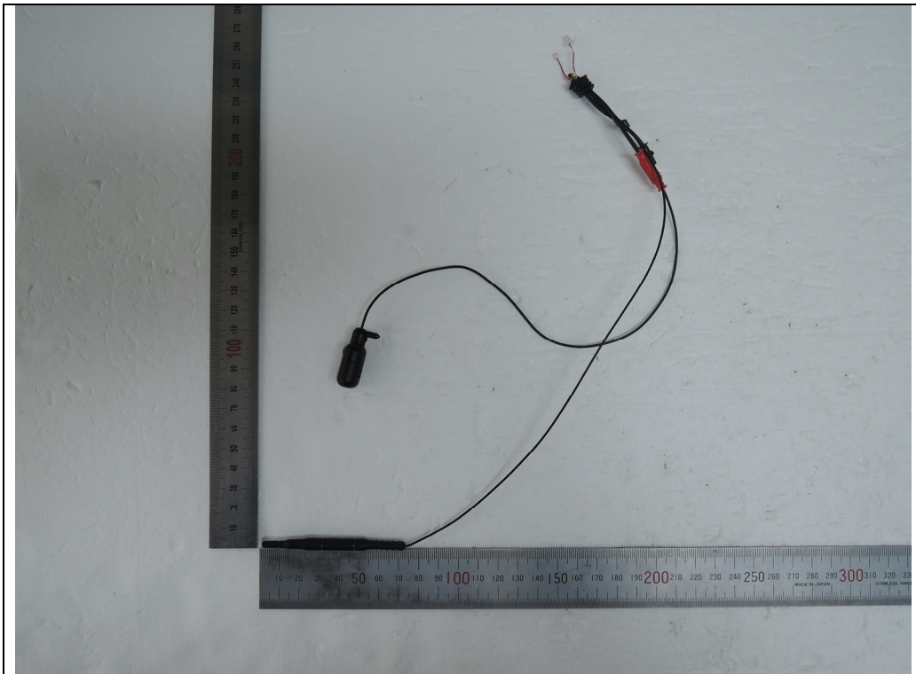
<Antenna_1>
