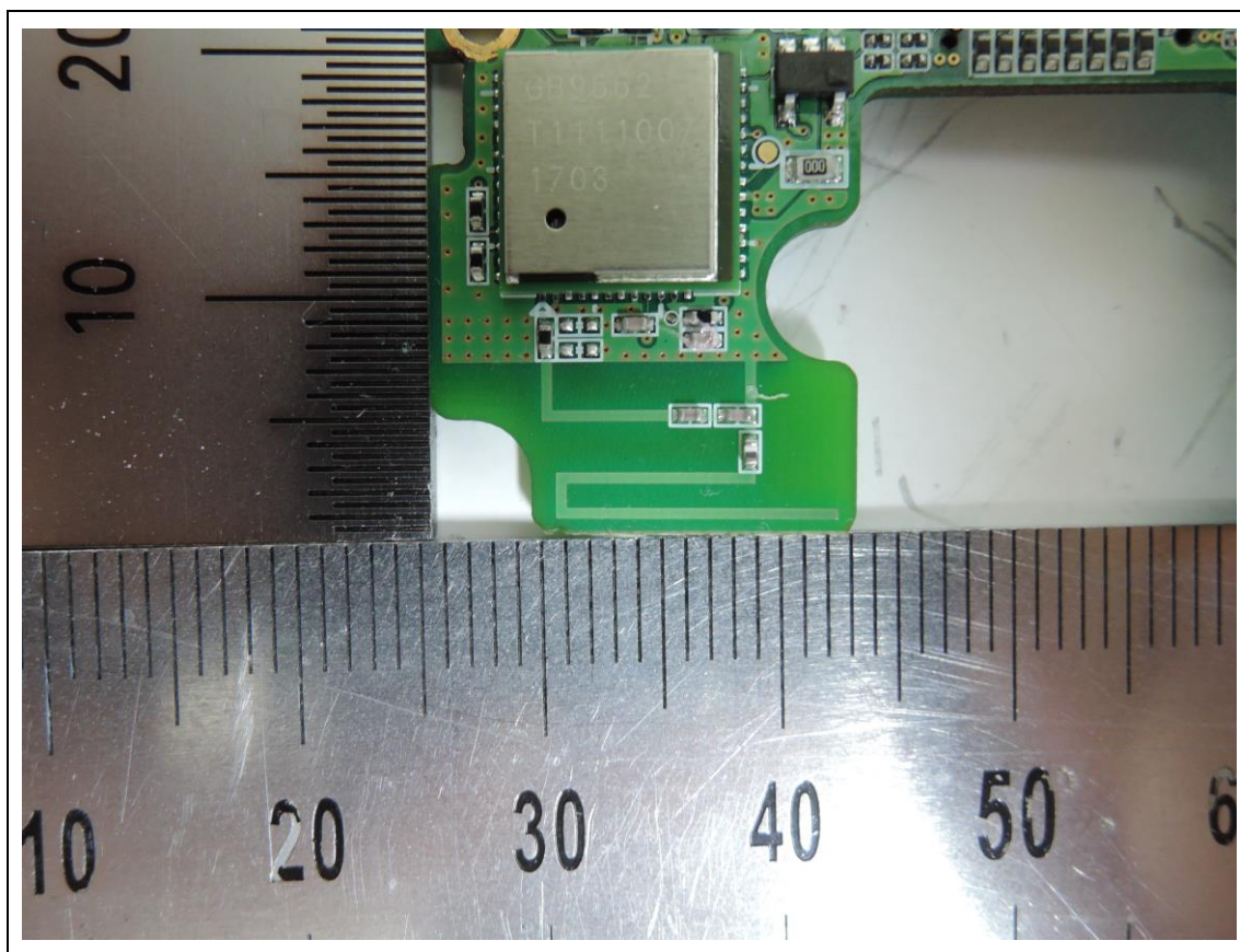
<Antenna>
