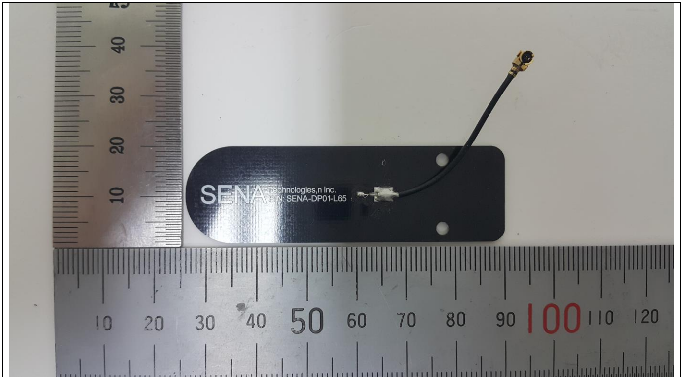
<Antenna 3>
