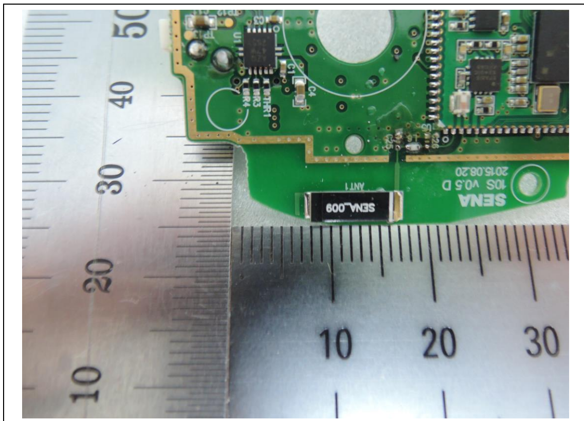
<Antenna>
