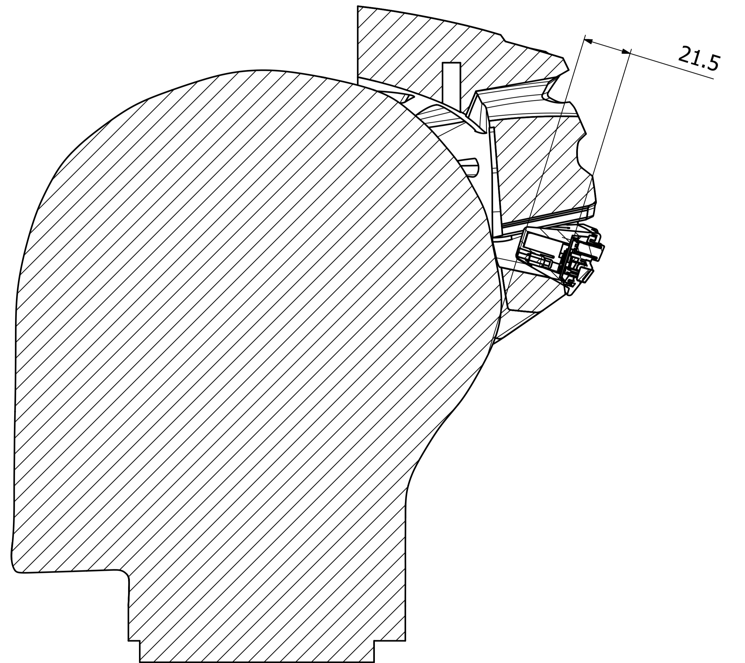
SECTION A-A
