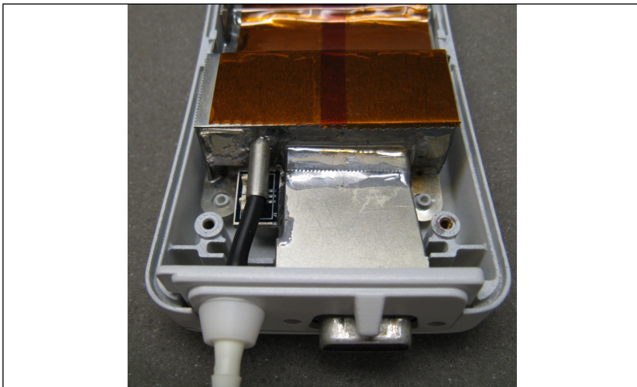
wSpO2 – Top (Zoomed In)
