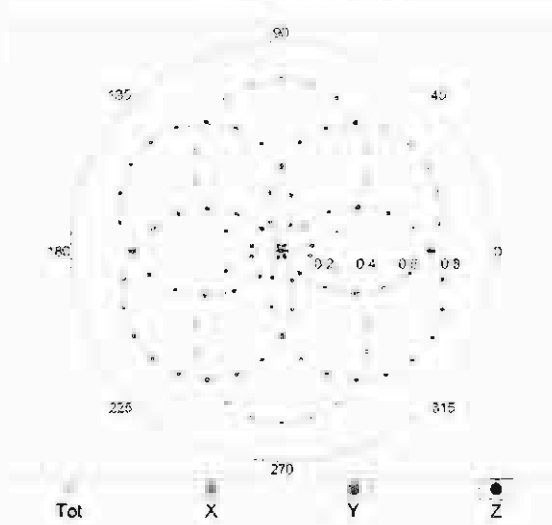
f=1800 MHz,R22
