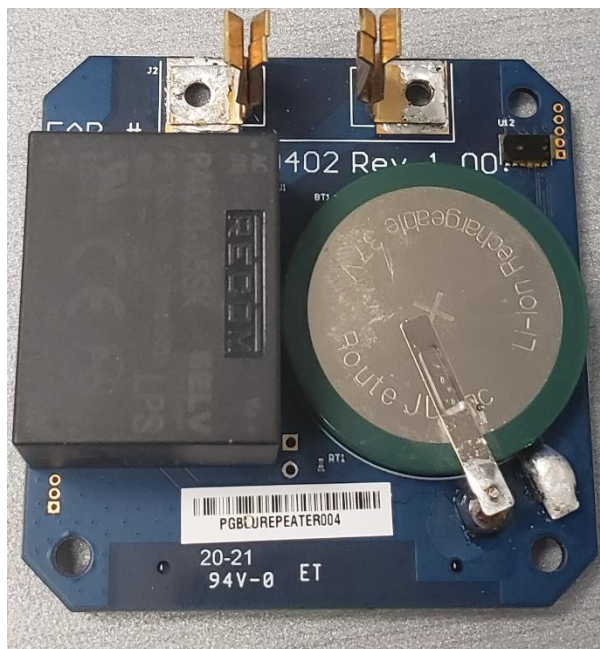
Bottom of BLUrepeater V1 PCB
