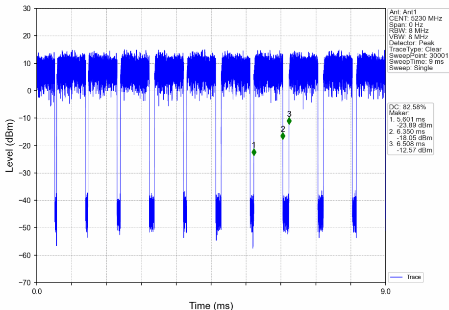
802.11ax(HEW40)_HCH_5230MHz_RU484_Left_Ant1_NTNV
