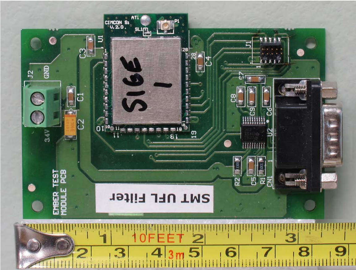
Front - UFL Antenna
