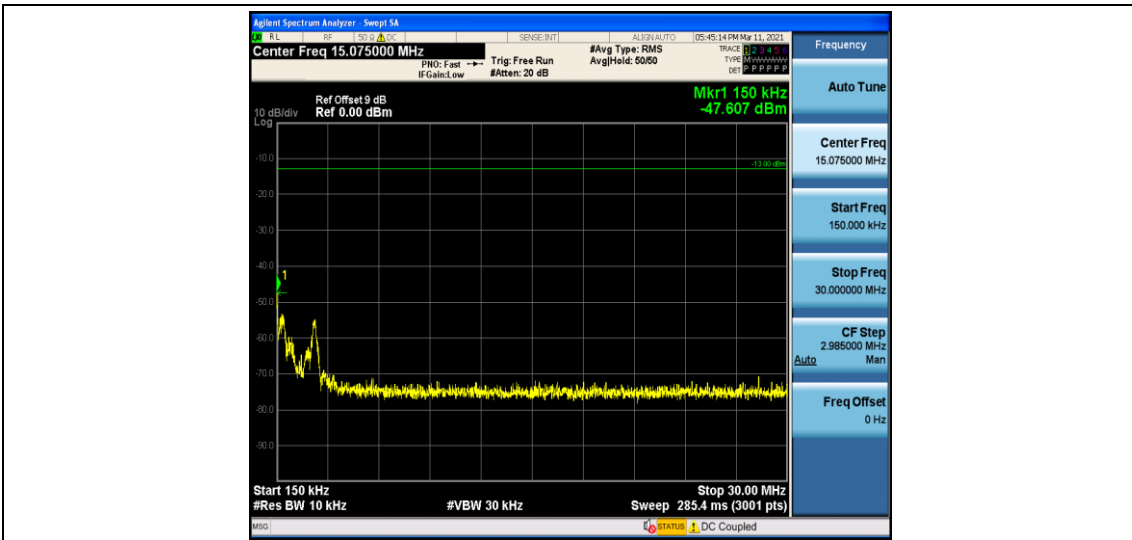
Band 71_10MHz_QPSK_133172_1RB#0
