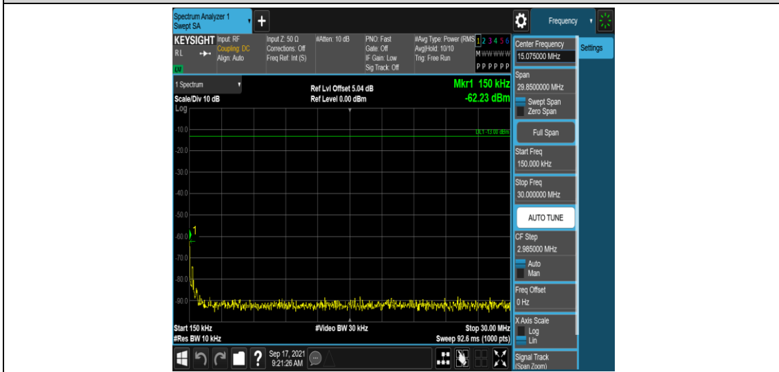
Band71-5MHz-QPSK-133297-1RB#0-Range2:0.15~30MHz
