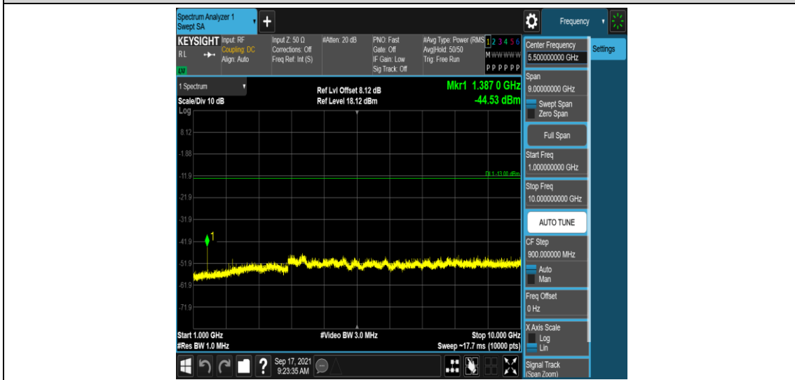
Band71-5MHz-QPSK-133447-1RB#0-Range4:1000~10000MHz
