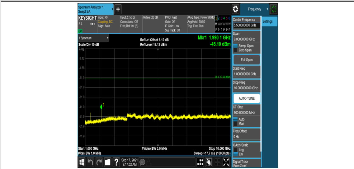
Band71-5MHz-QPSK-133147-1RB#0-Range4:1000~10000MHz
