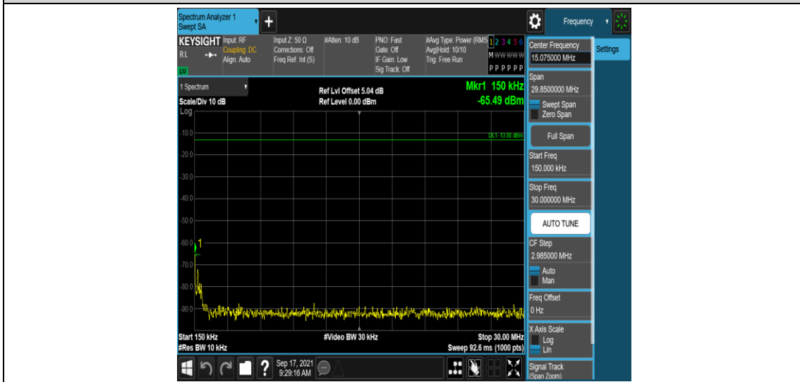
Band71-10MHz-QPSK-133297-1RB#0-Range2:0.15~30MHz
