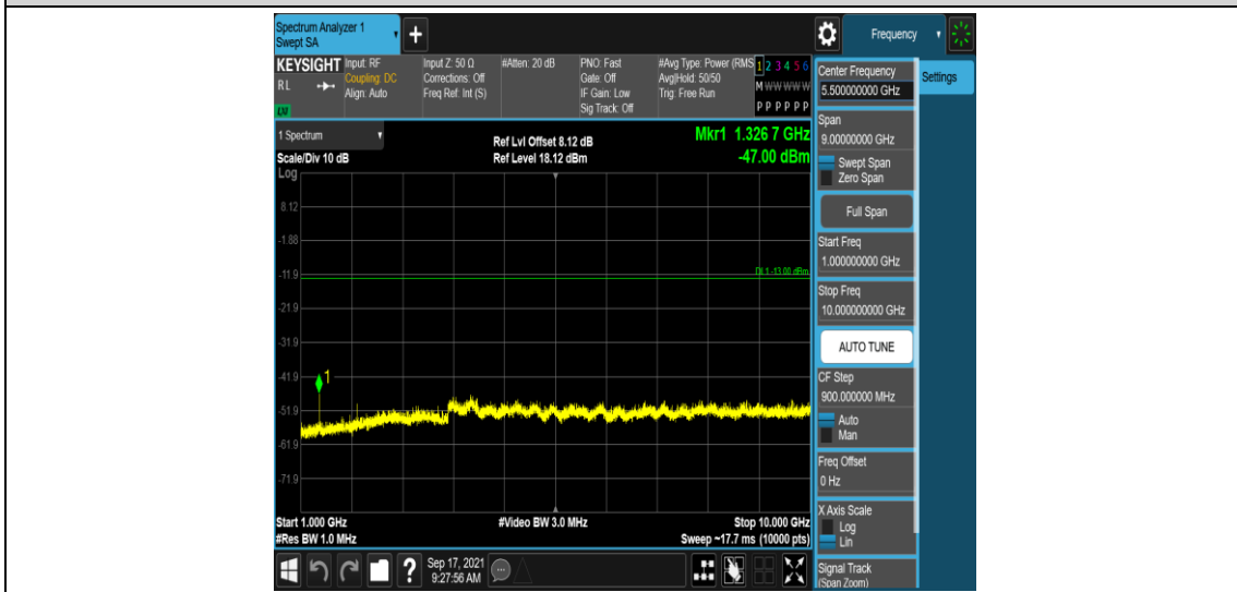
Band71-10MHz-QPSK-133172-1RB#0-Range4:1000~10000MHz
