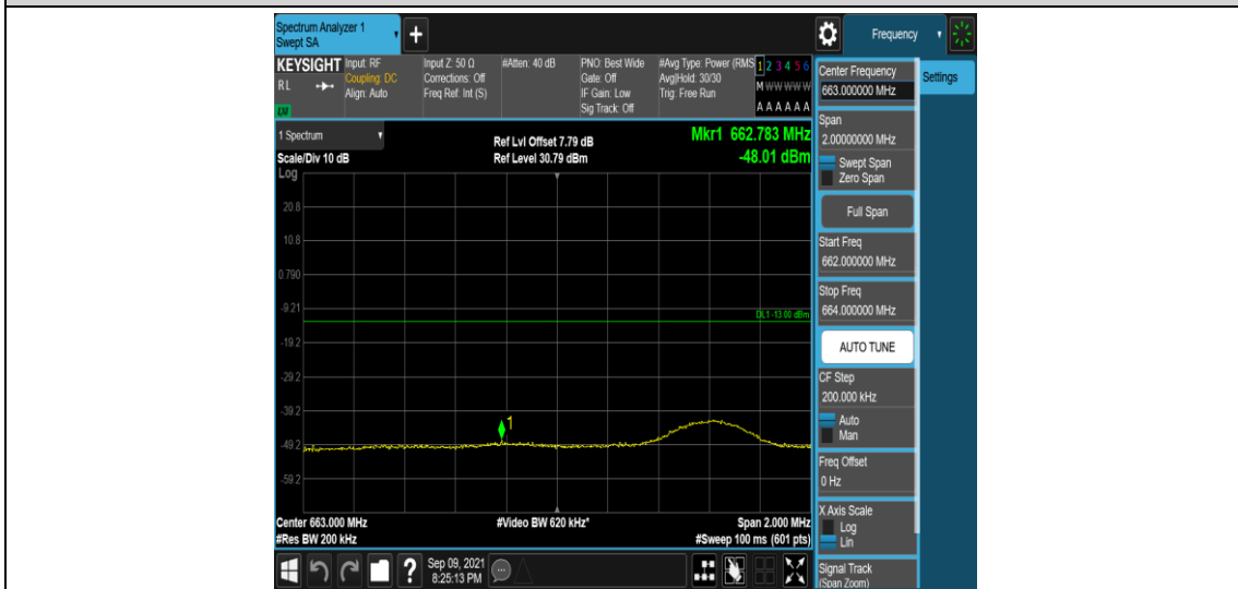
Band71-10MHz-QPSK-133172-1RB#49
