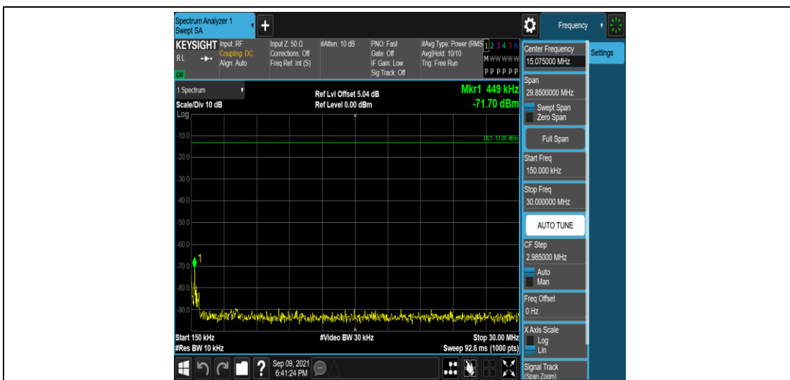
Band66-5MHz-QPSK-131997-1RB#0-Range2:0.15~30MHz
