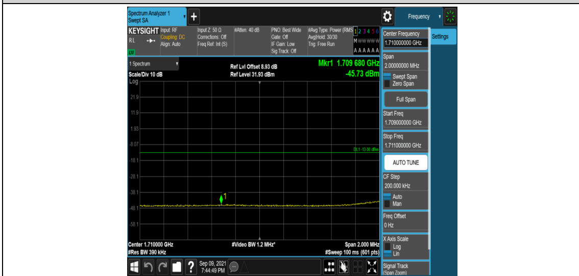
Band66-20MHz-QPSK-132072-1RB#99
