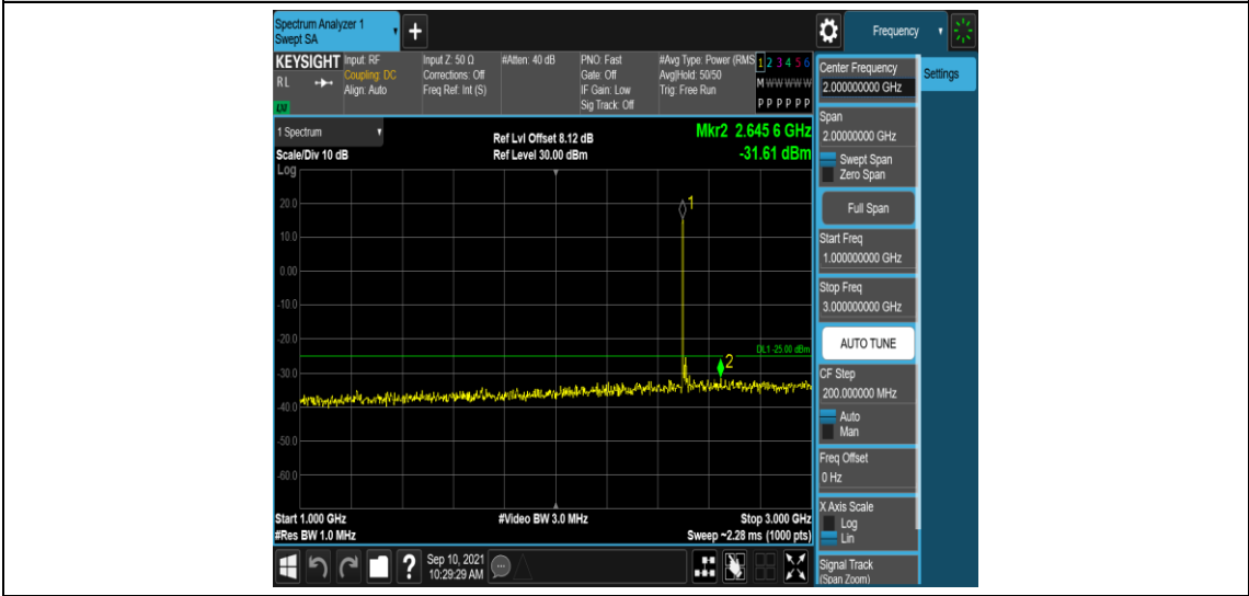
Band41-15MHz-QPSK-39725-1RB#0-Range4:1000~3000MHz
