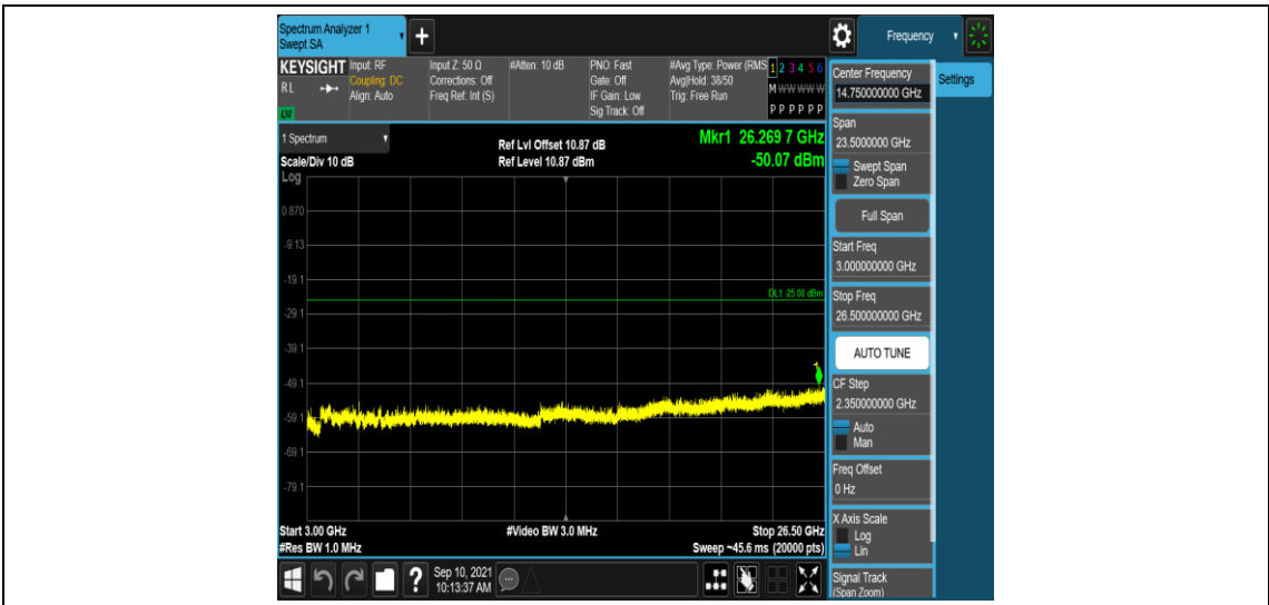
Band41-10MHz-QPSK-41540-1RB#0-Range5:3000~26500MHz
