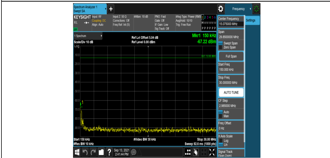
Band26-5MHz-QPSK-27015-1RB#0-Range2:0.15~30MHz
