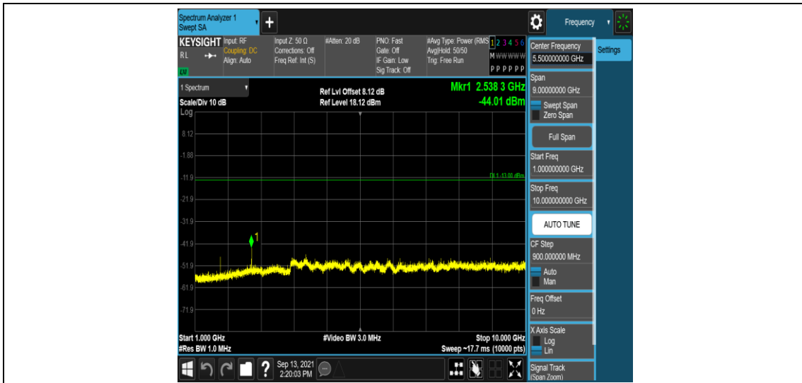
Band26-3MHz-QPSK-27025-1RB#0-Range4:1000~10000MHz
