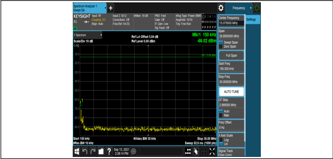
Band26-5MHz-QPSK-26815-1RB#0-Range2:0.15~30MHz
