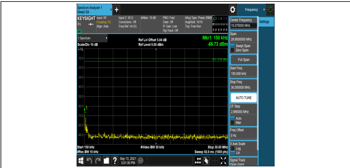
Band26-10MHz-QPSK-26915-1RB#0-Range2:0.15~30MHz
