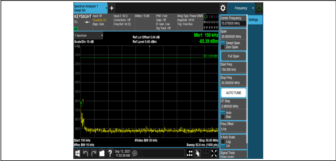
Band26-10MHz-QPSK-26740-1RB#0-Range2:0.15~30MHz
