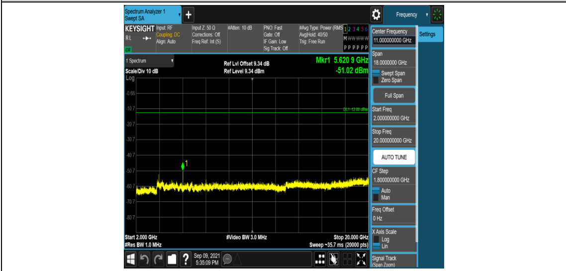
Band25-20MHz-QPSK-26365-1RB#0-Range5:2000~20000MHz
