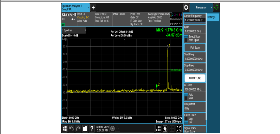
Band25-20MHz-QPSK-26365-1RB#0-Range4:1000~2000MHz
