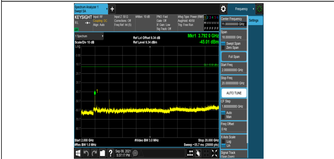
Band25-20MHz-QPSK-26590-1RB#0-Range5:2000~20000MHz
