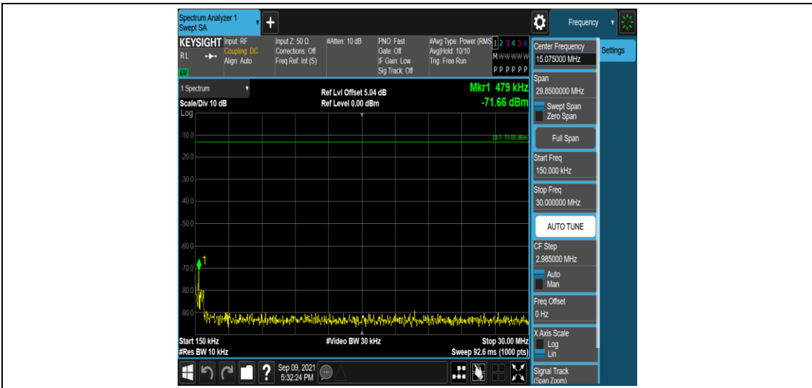
Band25-20MHz-QPSK-26140-1RB#0-Range2:0.15~30MHz
