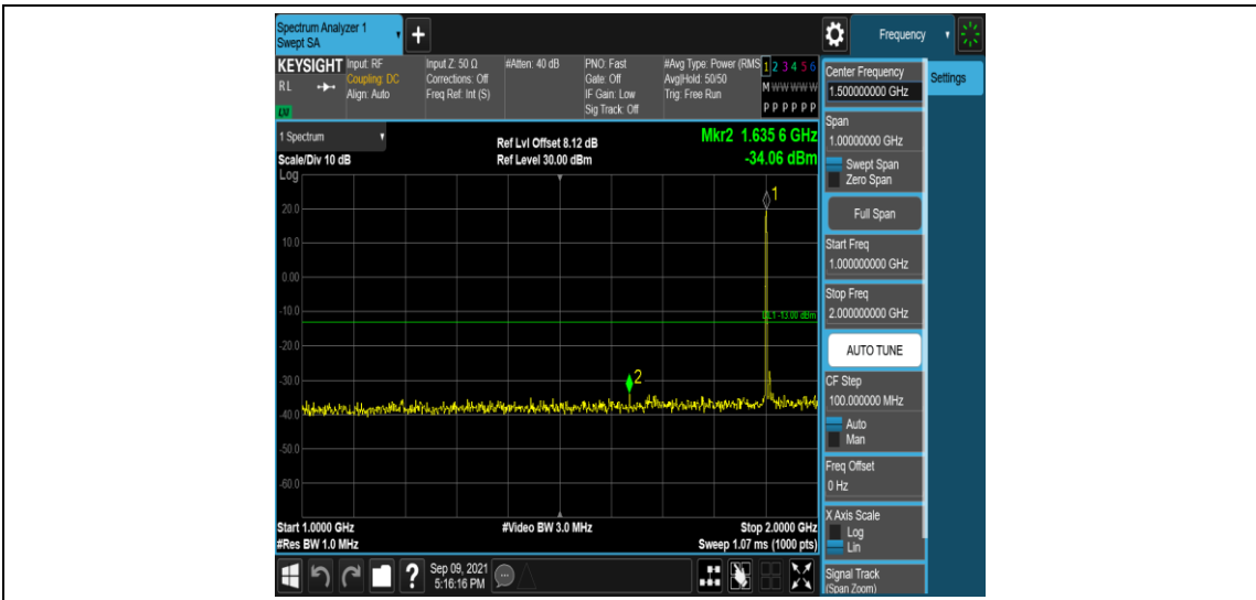
Band25-15MHz-QPSK-26615-1RB#0-Range4:1000~2000MHz
