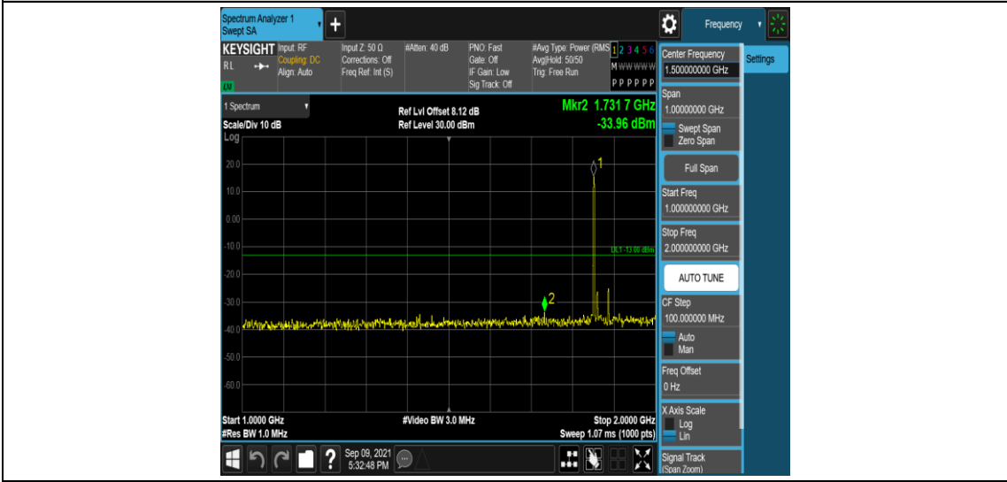
Band25-20MHz-QPSK-26140-1RB#0-Range4:1000~2000MHz
