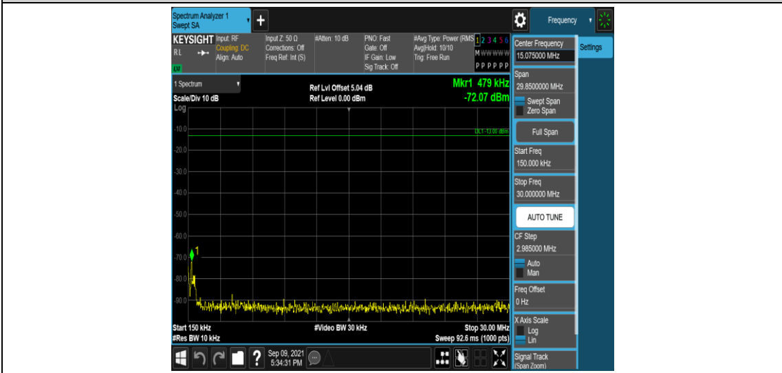
Band25-20MHz-QPSK-26365-1RB#0-Range2:0.15~30MHz
