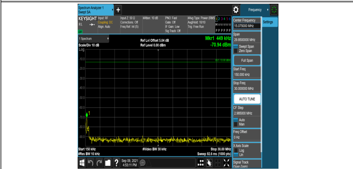
Band25-10MHz-QPSK-26365-1RB#0-Range2:0.15~30MHz
