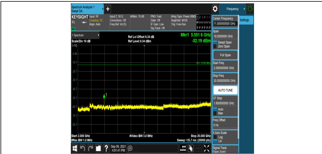
Band25-10MHz-QPSK-26090-1RB#0-Range5:2000~20000MHz
