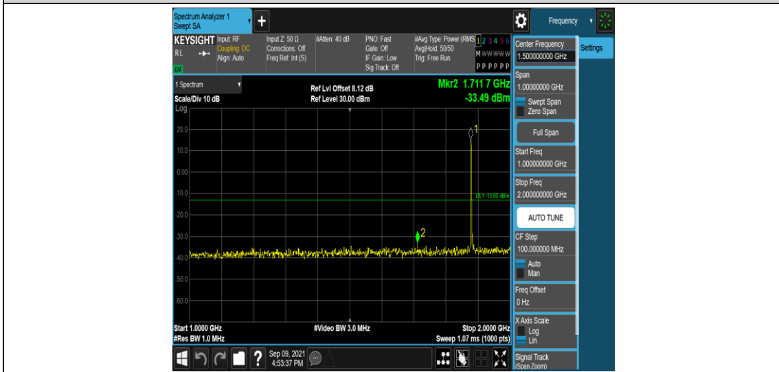
Band25-10MHz-QPSK-26365-1RB#0-Range4:1000~2000MHz
