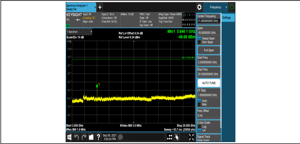
Band25-1.4MHz-QPSK-26365-1RB#0-Range5:2000~20000MHz
