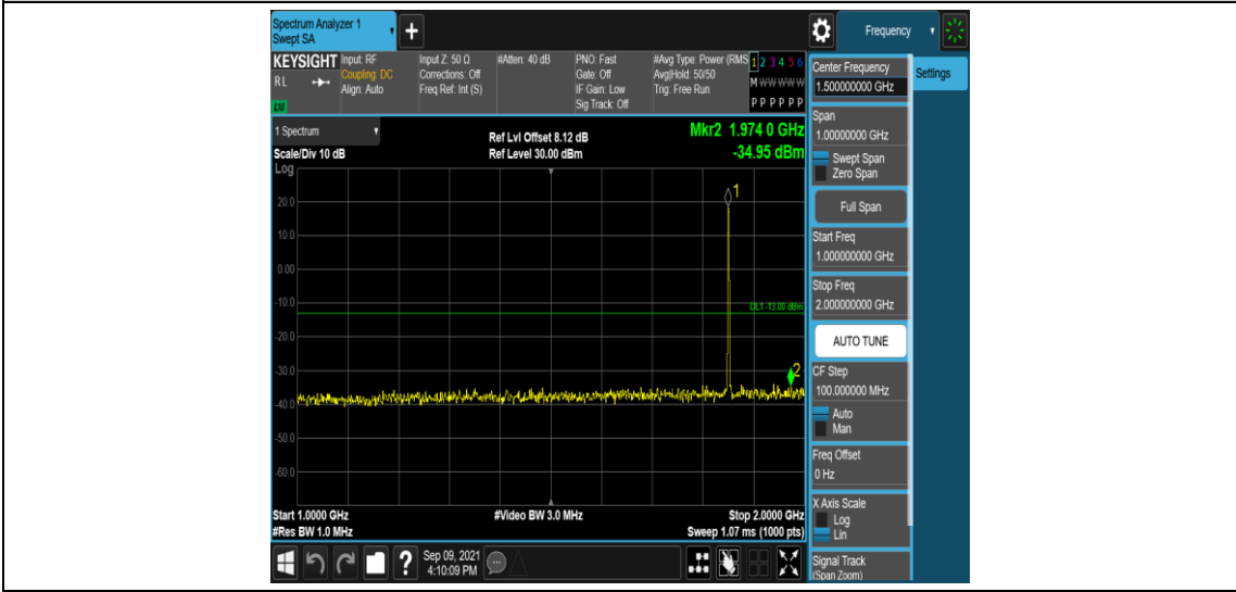
Band25-3MHz-QPSK-26055-1RB#0-Range4:1000~2000MHz
