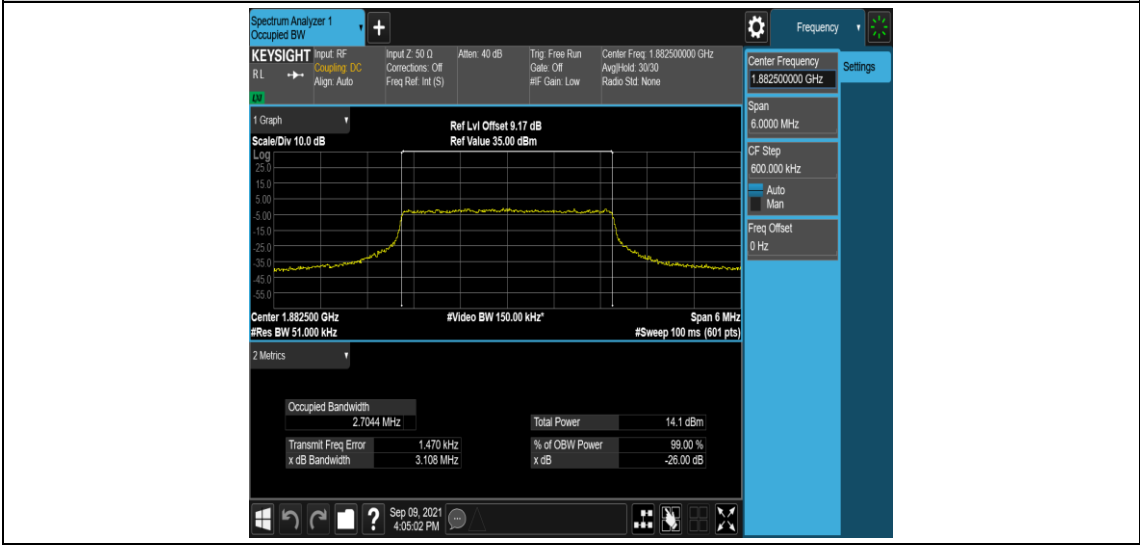
Band25-3MHz-QPSK-26365-15RB#0
