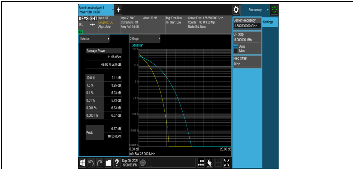
Band25-10MHz-QPSK-26365-50RB#0
