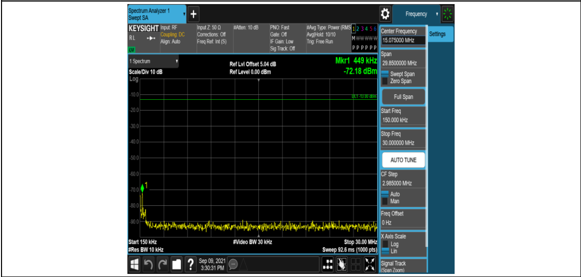
Band4-20MHz-QPSK-20300-1RB#0-Range2:0.15~30MHz
