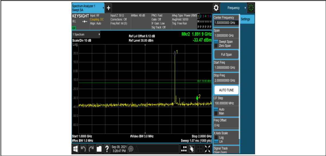
Band4-20MHz-QPSK-20175-1RB#0-Range4:1000~2000MHz
