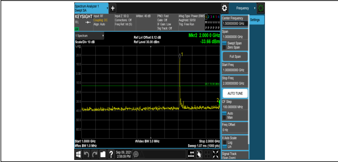
Band4-15MHz-QPSK-2025-1RB#0-Range4:1000~2000MHz
