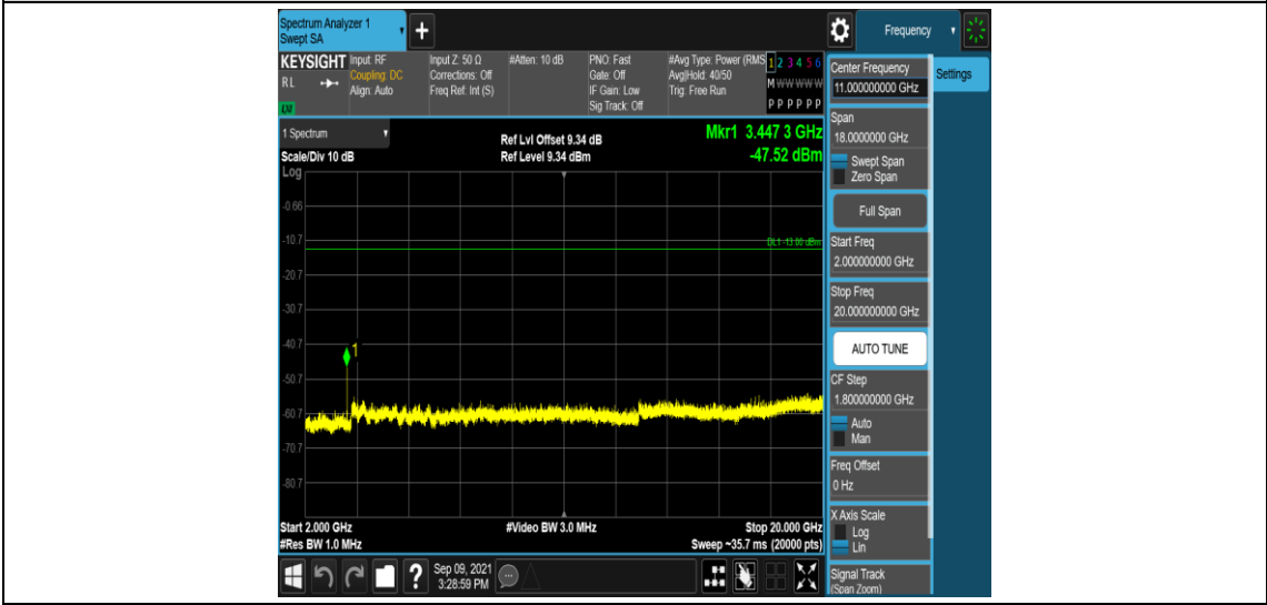
Band4-20MHz-QPSK-20175-1RB#0-Range5:2000~20000MHz
