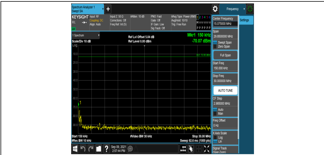
Band4-15MHz-QPSK-2025-1RB#0-Range2:0.15~30MHz
