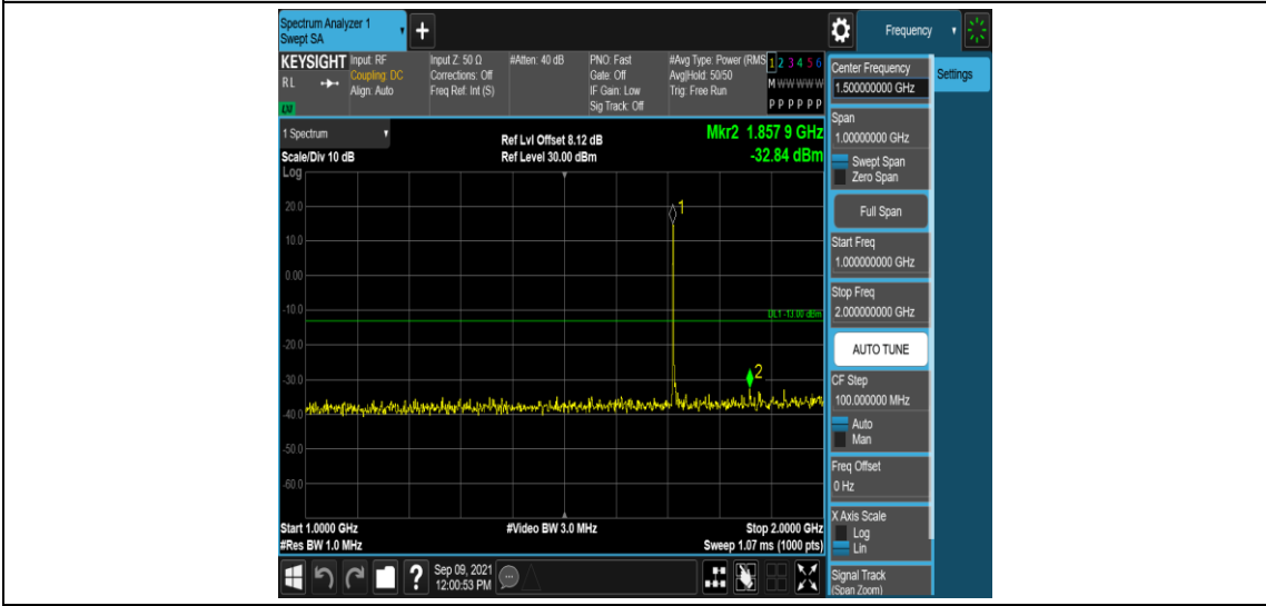
Band4-5MHz-QPSK-19975-1RB#0-Range4:1000~2000MHz
