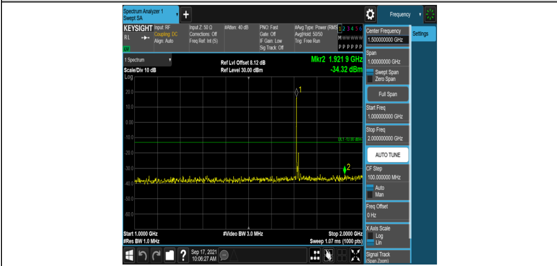
Band4-10MHz-QPSK-20000-1RB#0-Range4:1000~2000MHz
