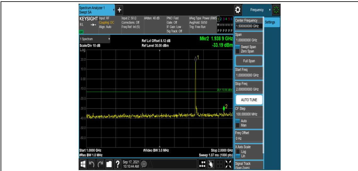
Band4-10MHz-QPSK-20350-1RB#0-Range4:1000~2000MHz
