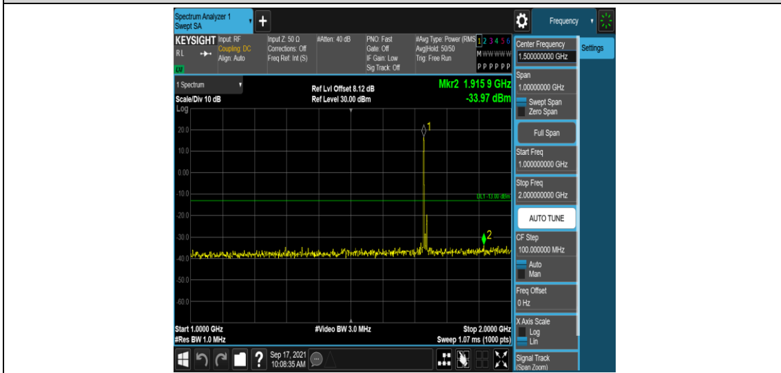
Band4-10MHz-QPSK-20175-1RB#0-Range4:1000~2000MHz
