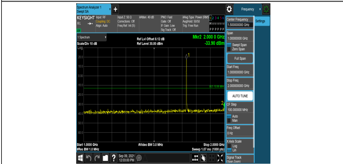
Band4-5MHz-QPSK-20175-1RB#0-Range4:1000~2000MHz
