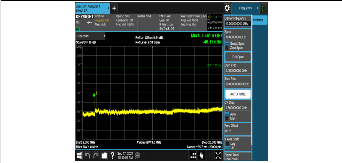
Band4-10MHz-QPSK-20350-1RB#0-Range5:2000~20000MHz
