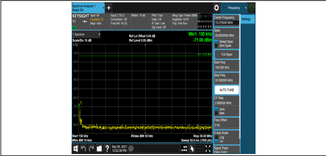
Band4-5MHz-QPSK-20175-1RB#0-Range2:0.15~30MHz
