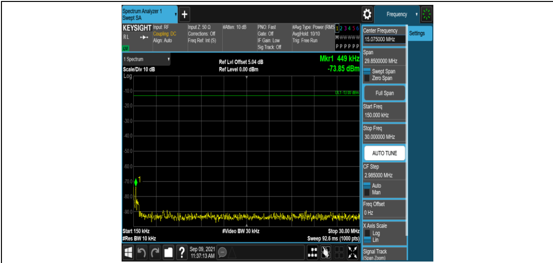
Band4-3MHz-QPSK-19965-1RB#0-Range2:0.15~30MHz
