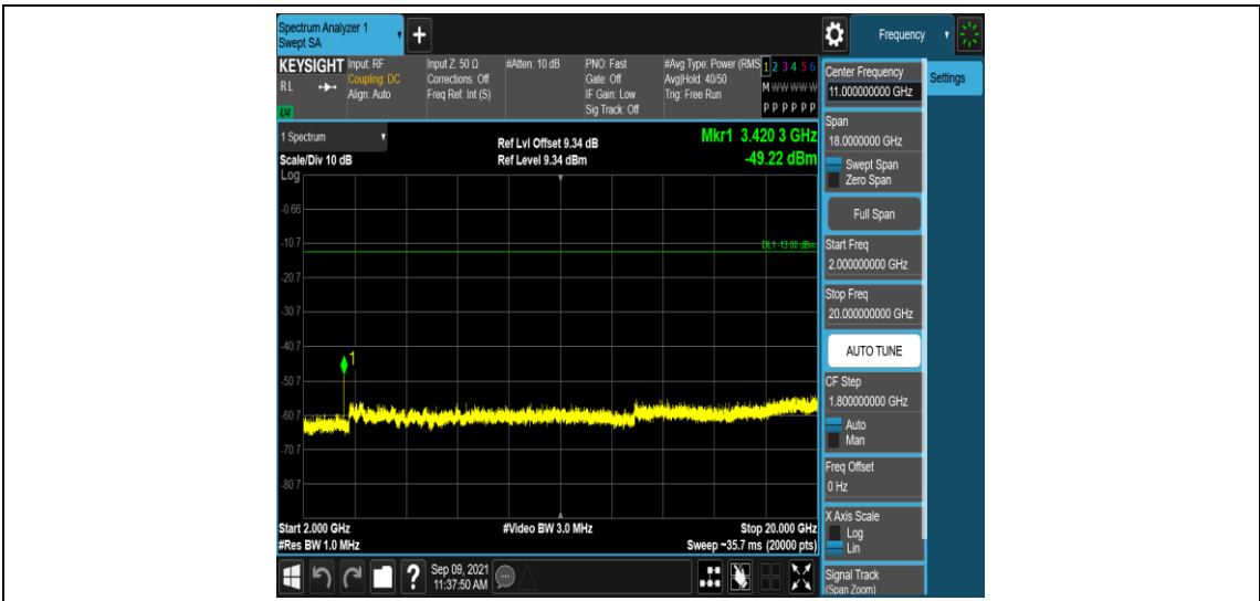
Band4-3MHz-QPSK-19965-1RB#0-Range5:2000~20000MHz
