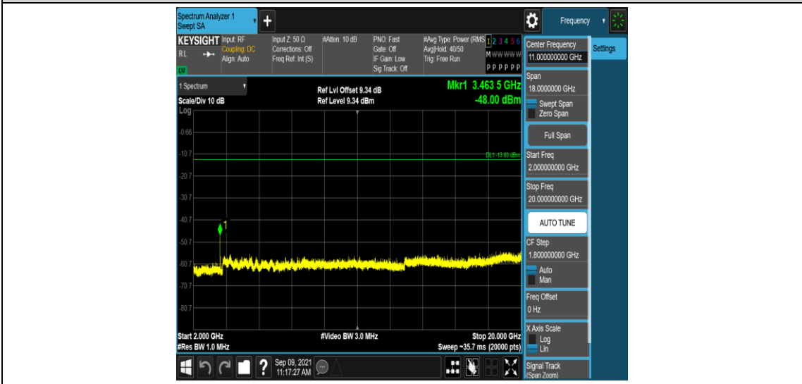
Band4-1.4MHz-QPSK-20175-1RB#0-Range5:2000~20000MHz
