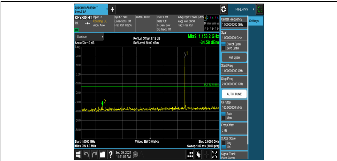
Band4-3MHz-QPSK-20385-1RB#0-Range4: 1000~2000MHz
