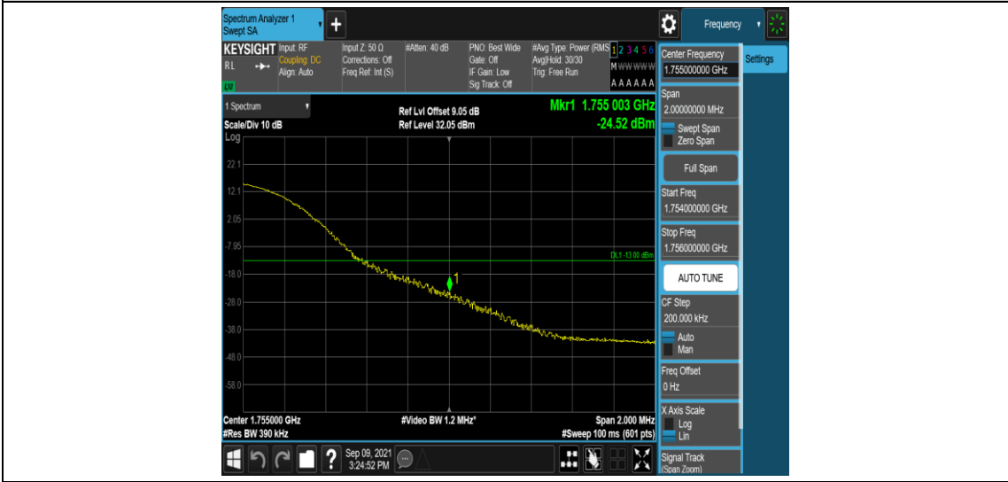
Band4-20MHz-QPSK-20300-1RB#99
