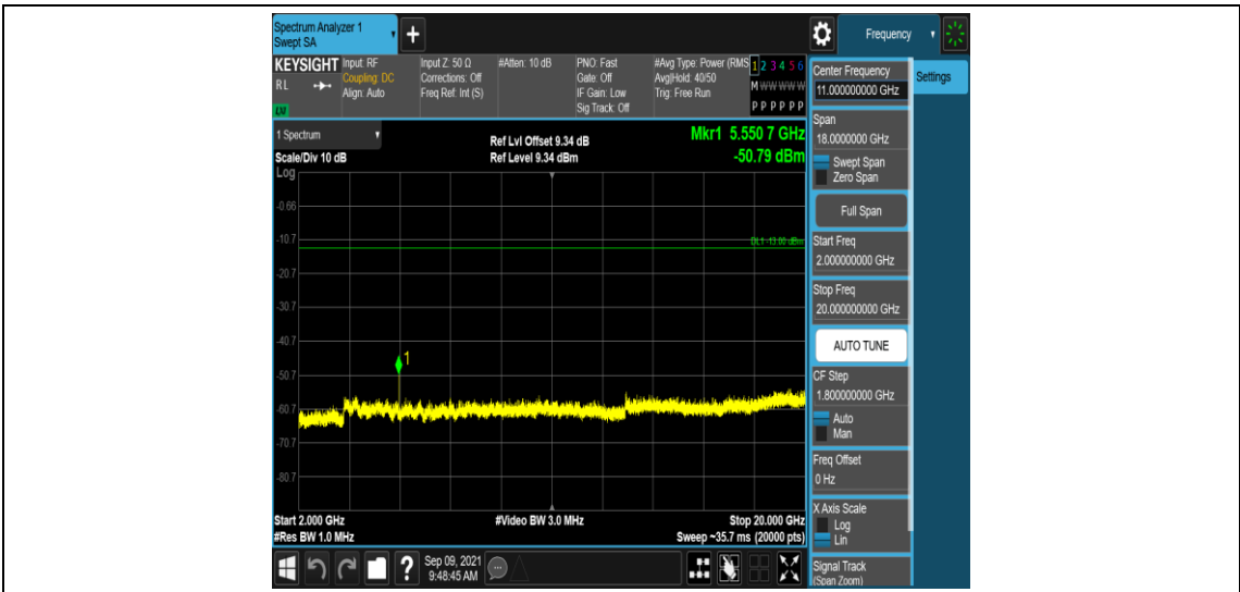
Band2-5MHz-QPSK-18625-1RB#0-Range5:2000~20000MHz
