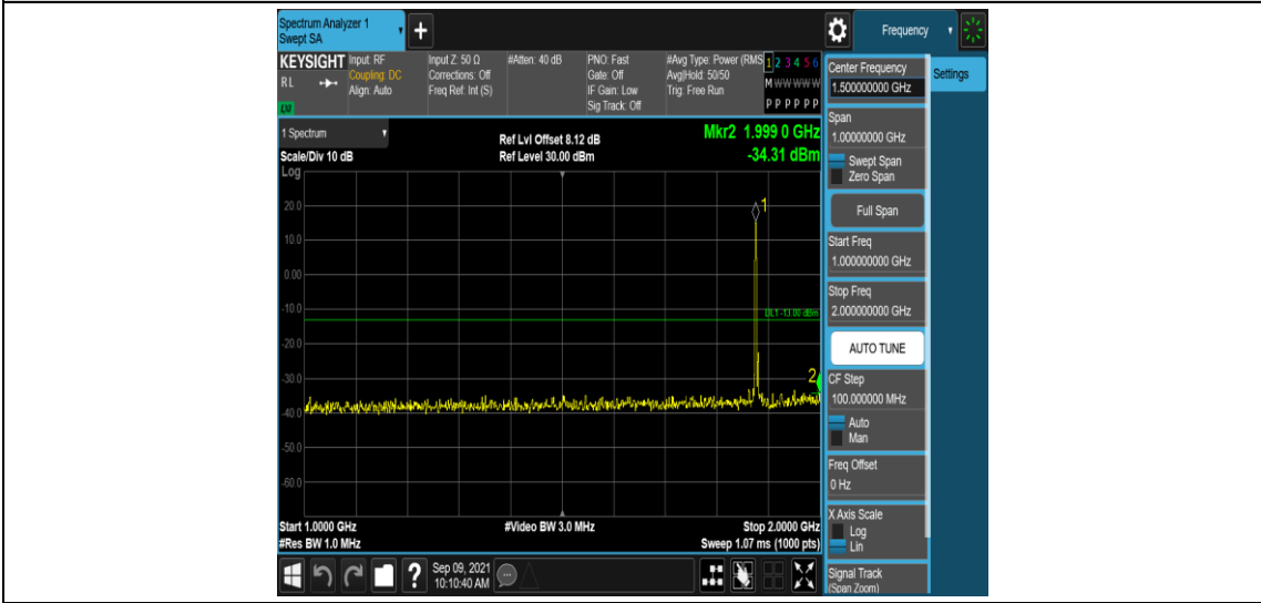
Band2-10MHz-QPSK-18900-1RB#0-Range4:1000~2000MHz
