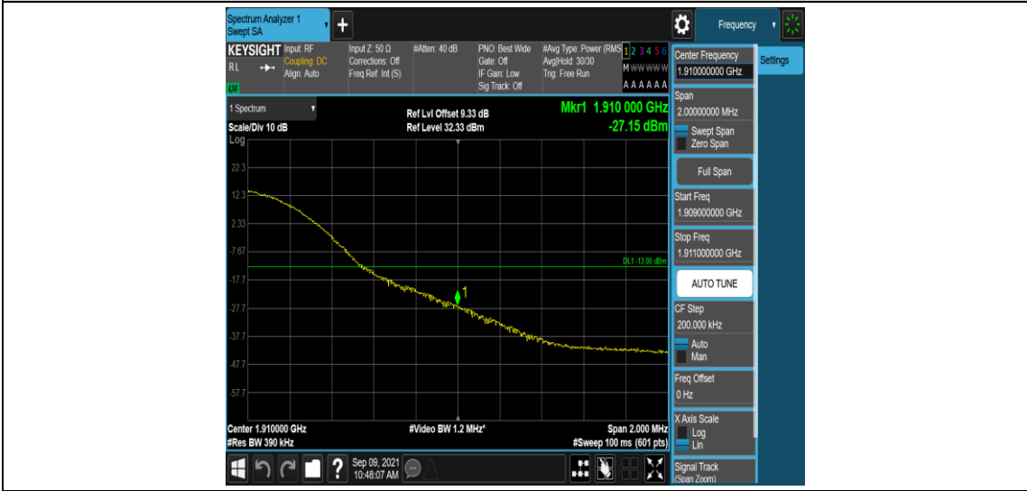
Band2-20MHz-16QAM-19100-1RB#90
