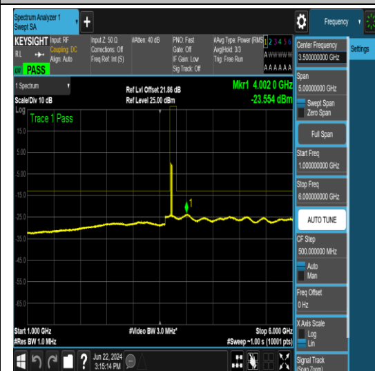
NTNV_N78-3700-3800_PC2_30_40_L_TID21_NS _01_18000_40000_#1
