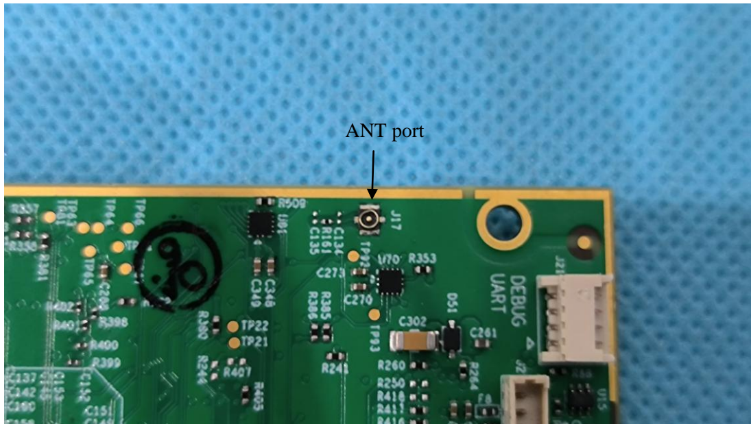
Antenna
