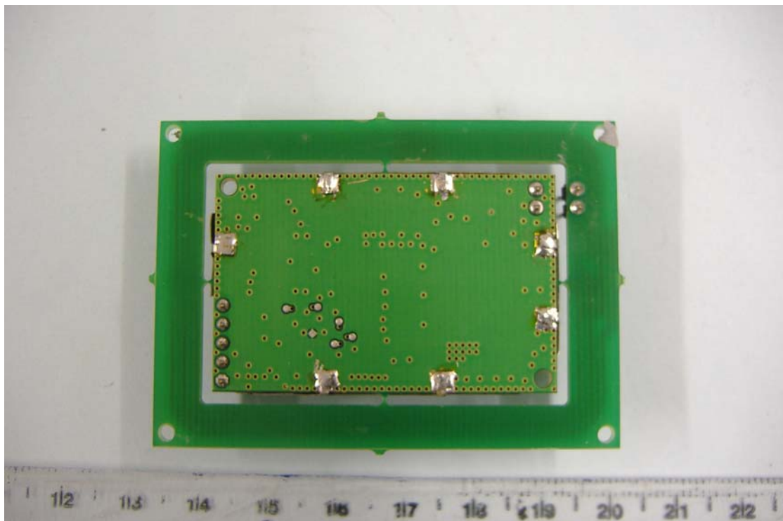
EUT BOTTOM OVERVIEW
