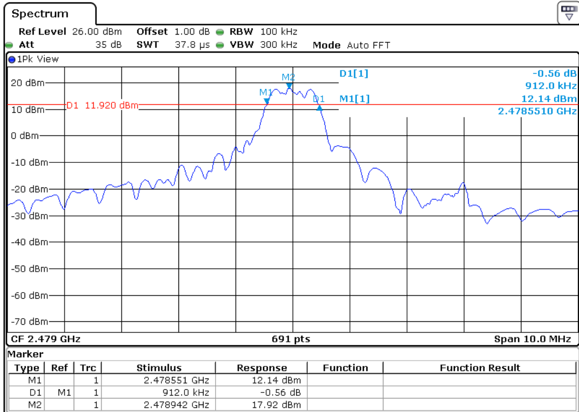
2.4GHz wireless module: BT-2405A
