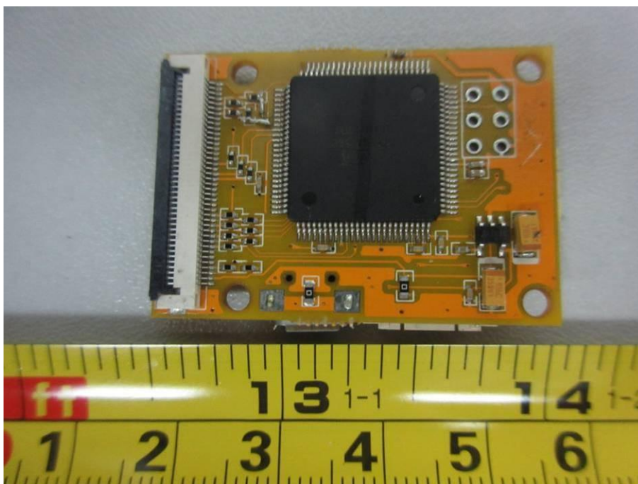
5.8G Transmitter Module
