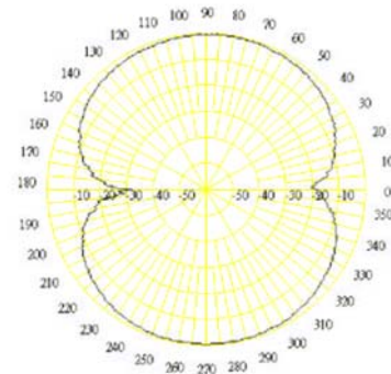
2.45-E-PLANE
