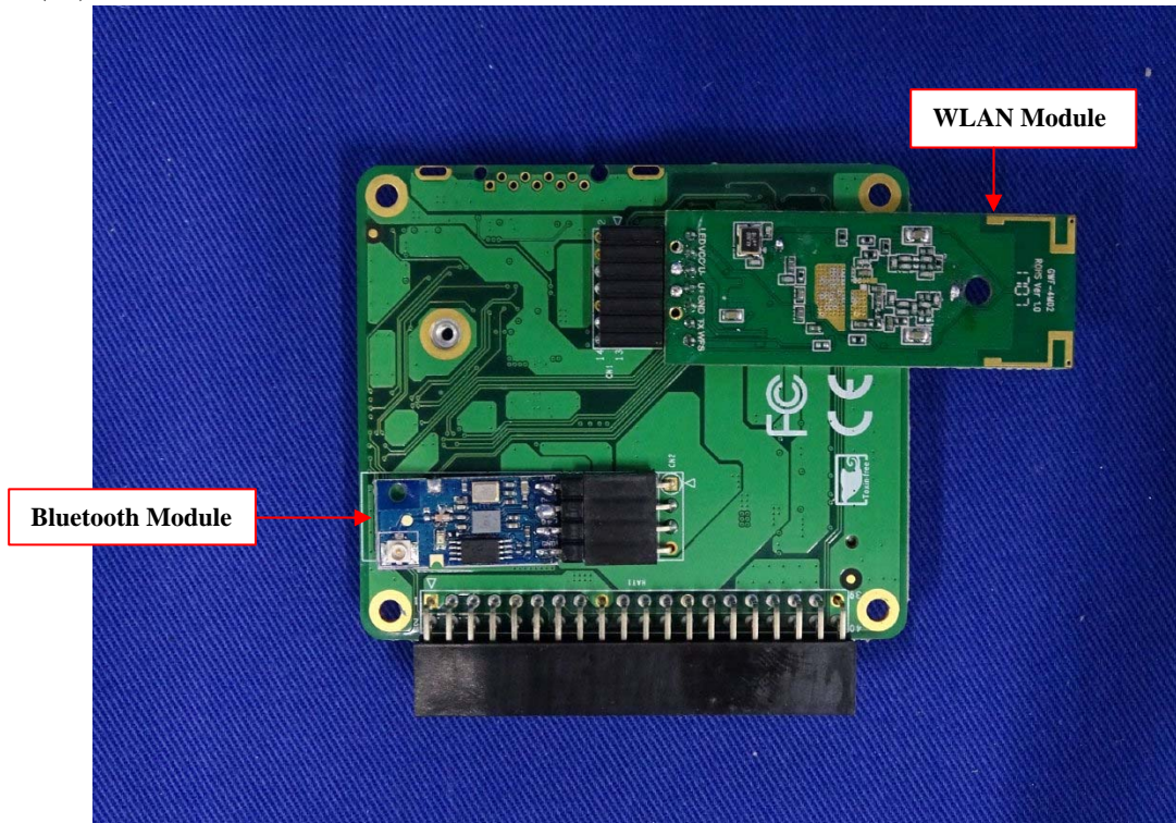
(12) EUT Photo
