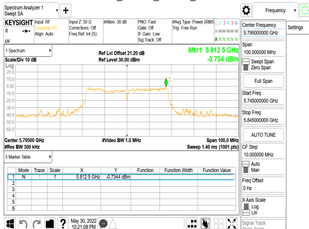
802.11ac_40MHz_Chain1_5795MHz
