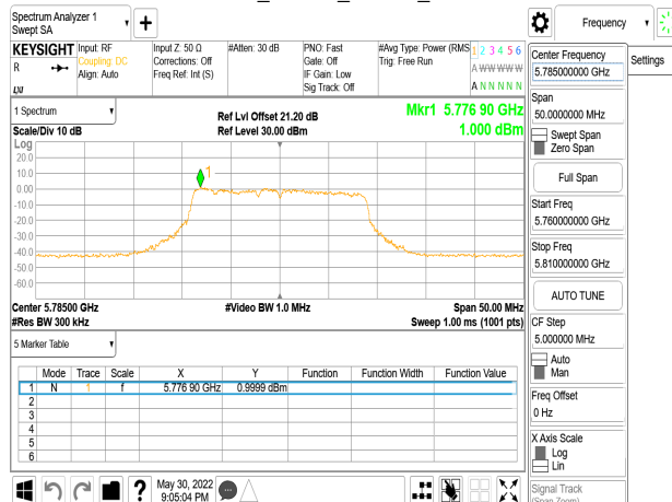
802.11ac_20MHz_Chain3_5785MHz
