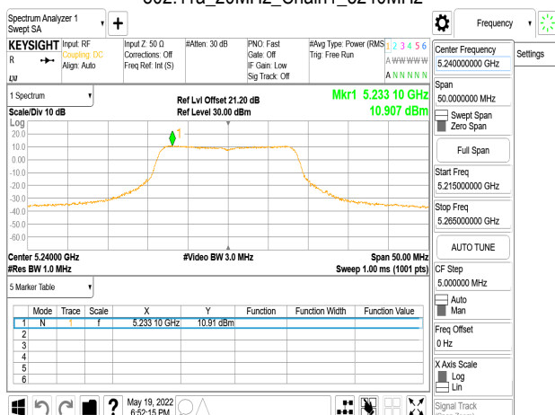
802.11a_20MHz_Chain1_5240MHz
