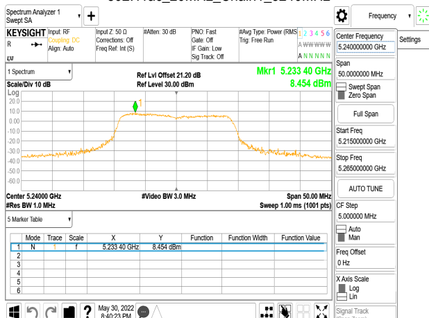
802.11ac_20MHz_Chain1_5240MHz
