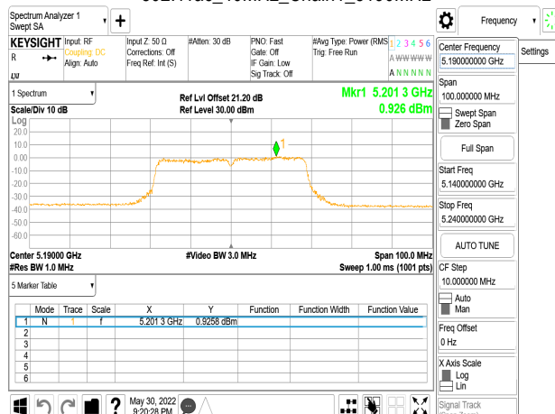
802.11ac_40MHz_Chain1_5190MHz
